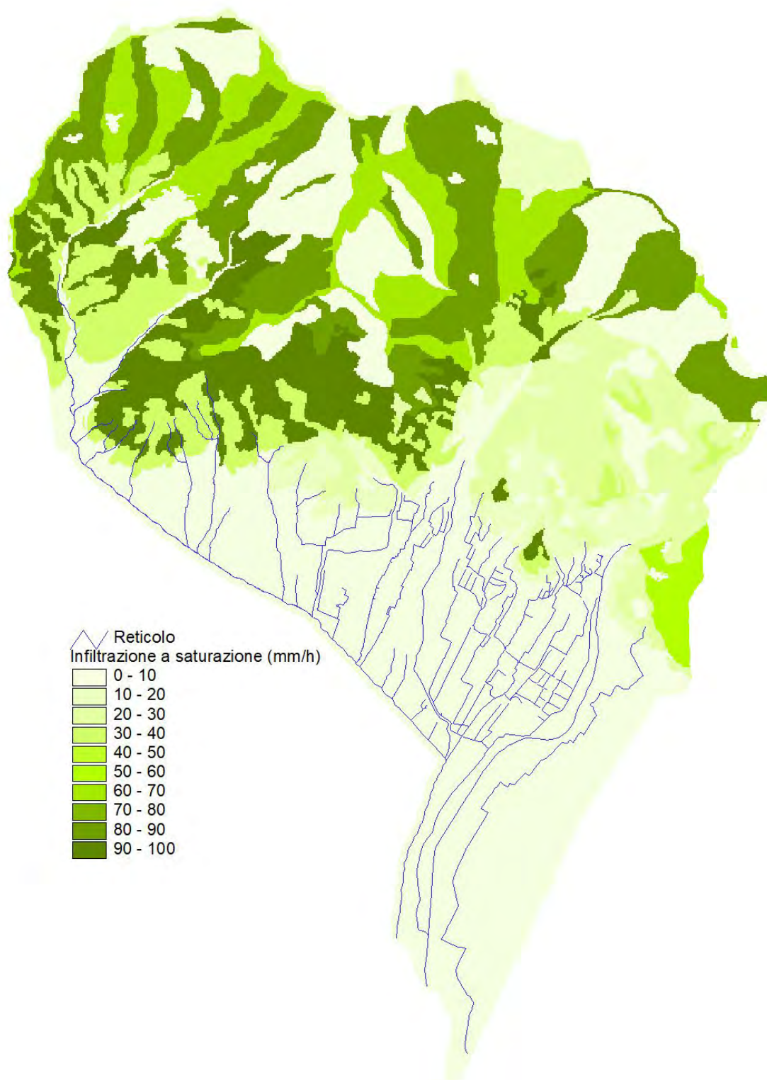
Figura 3-7 – Velocità filtrazione.
