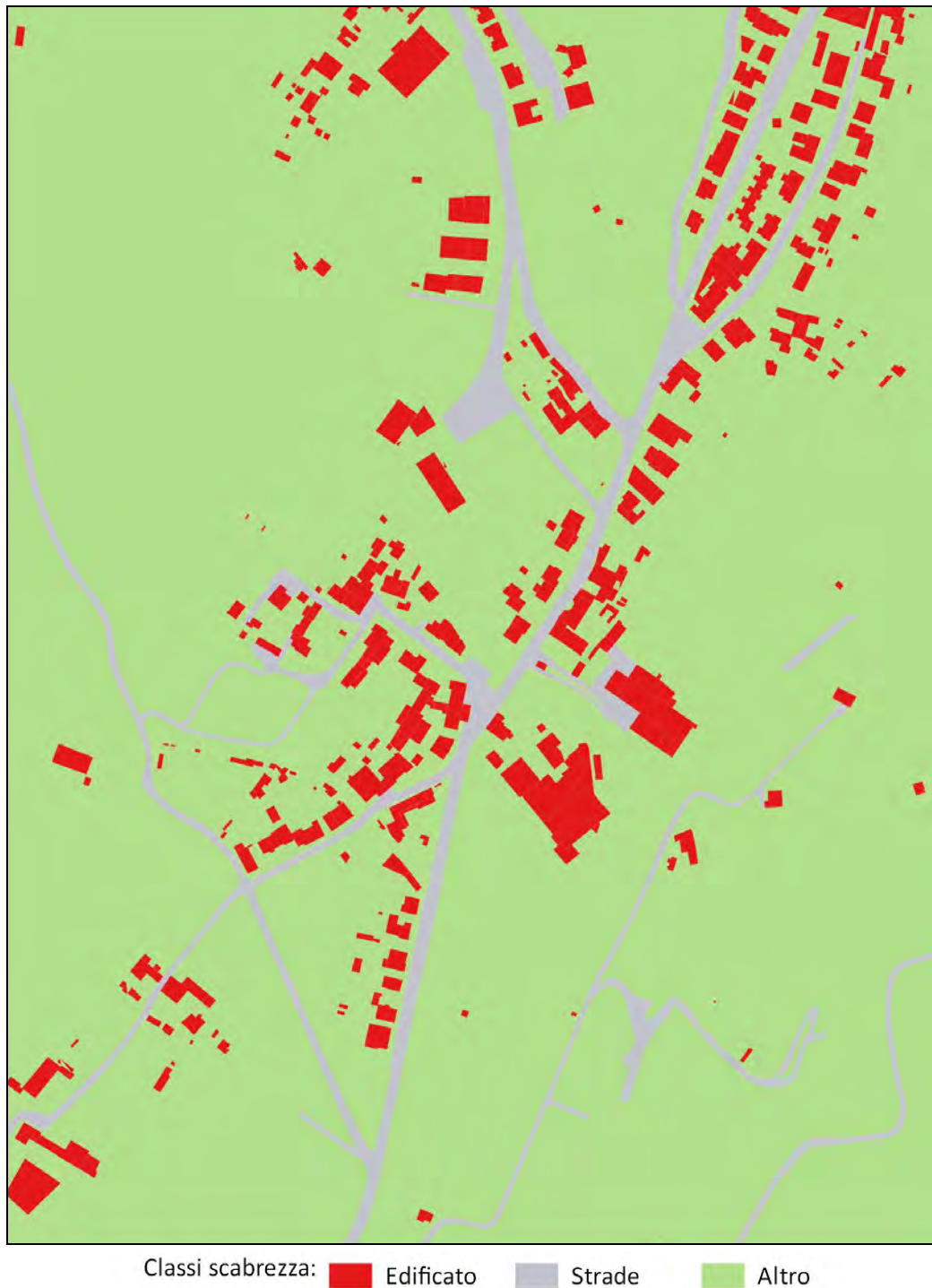
Figura 4-2 – Planimetria della copertura del suolo del modello bidimensionale (scala 1:5.000).
